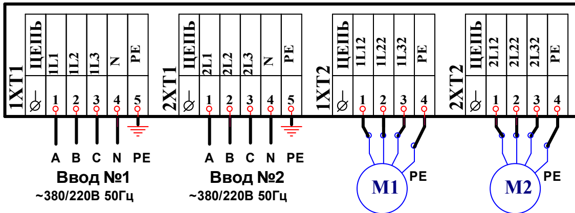
Схема подключения линий электропитания и двигателей
