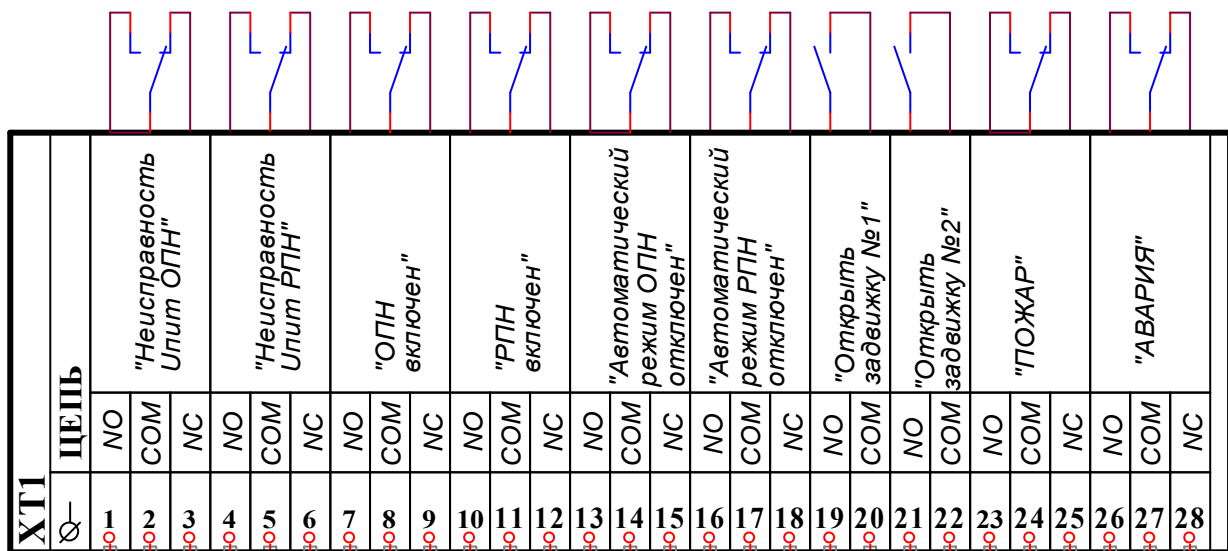
Схема формирования выходных сигналов (извещений)
